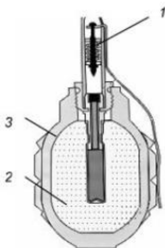
Hình 6-2. Cấu tạo lựu đạn \Phi 1
